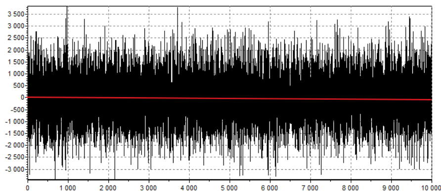
Рис. 10. Дробное броуновское движение. H=0.2 .
