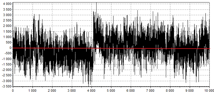
Рис. 9. Дробное броуновское движение. H=0.9 .
