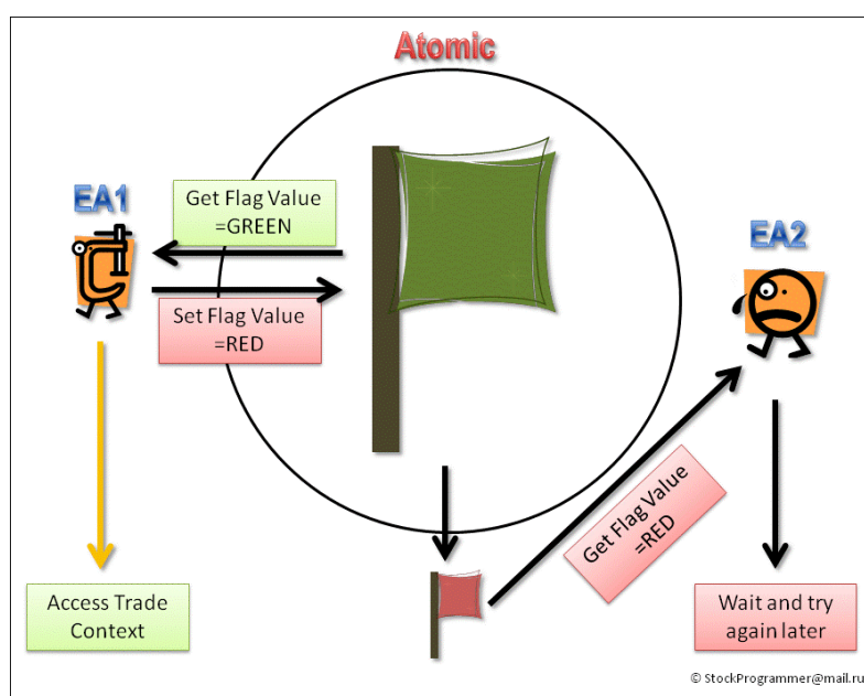
Рис. 4 - Атомарная операция
