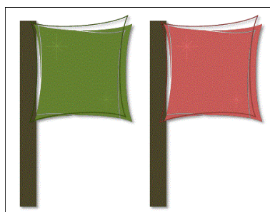
Рис. 1 - Семафор
