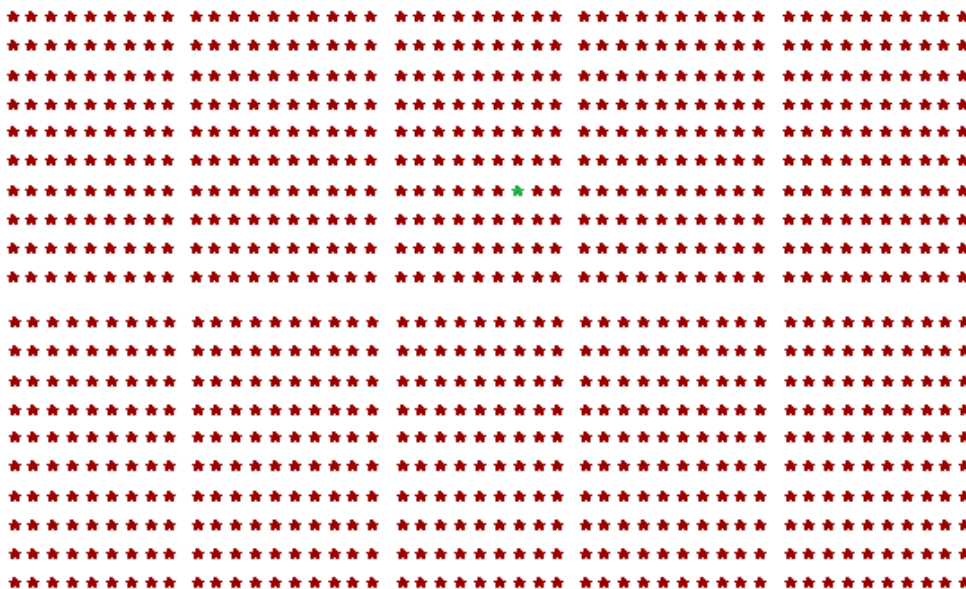
Рис. 1 - Иллюстрация вероятностей
