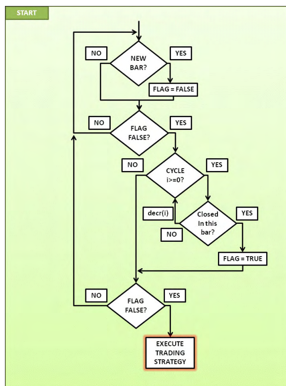
Рис. 1 – Алгоритм
