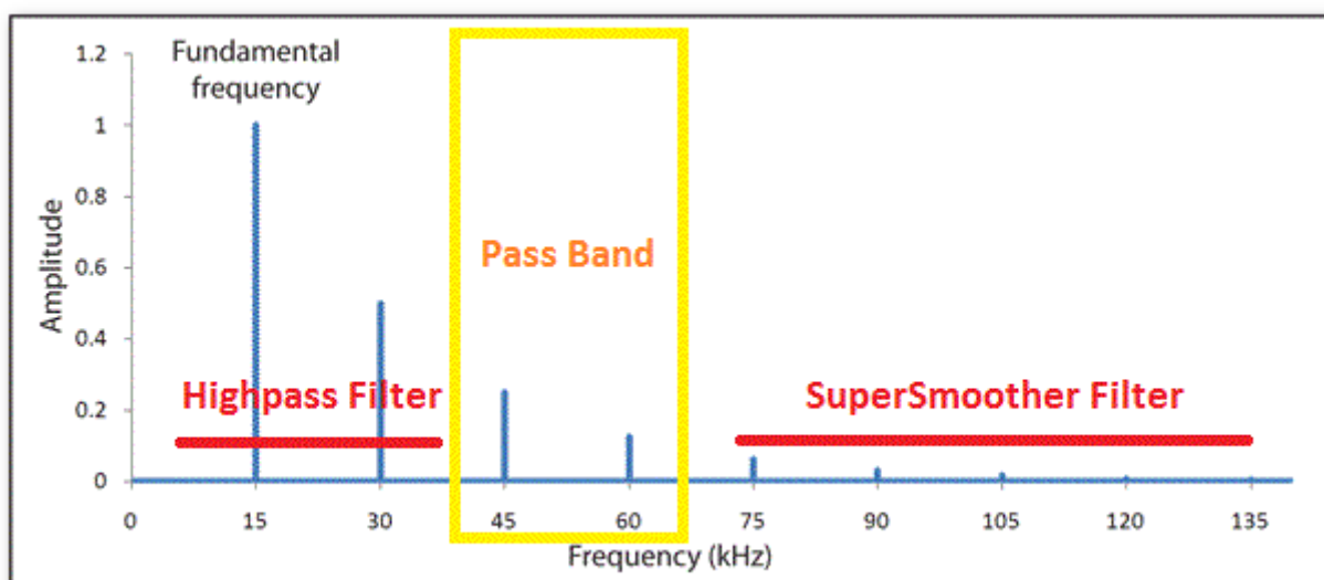
Рис.1 - Полоса частот
